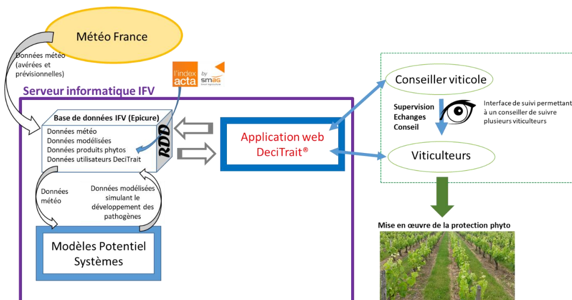
Figure 3. Fonctionnement des flux de données avec la version en ligne de DeciTrait. Functioning of the flows of data with the on-line version of DeciTrait
