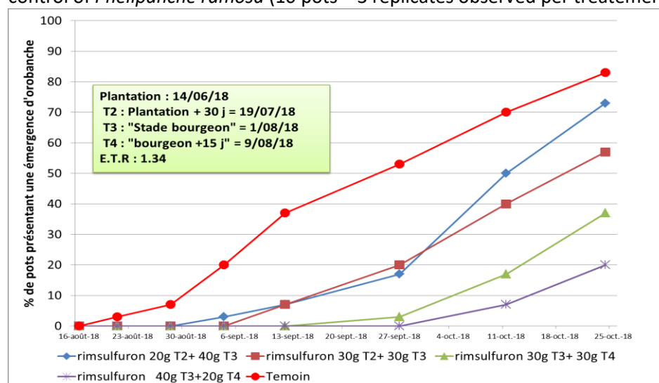
Figure 2 : 2018 — Effet du rimsulfuron sur le pourcentage de pots avec présence d’émergence d’orobanche rameuse (10 pots observés * 3 blocs par modalité) - 2018 - Effects of rimsulfuron on the control of Phelipanche ramosa (10 pots * 3 replicates observed per traitements)
